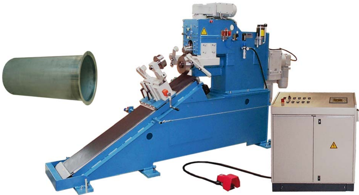
SME 200/4 P For rolling rings. Pour le cintrage d'anneaux.
